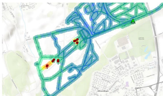
Figure 6 Exercice de recherche de sources radioactives avec un véhicule de radiométrie
